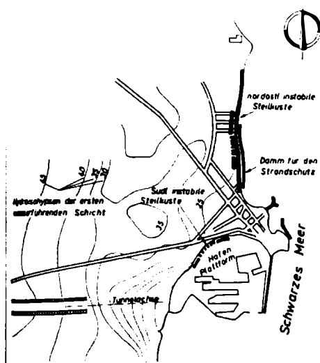
Fig. 1 – Situație falezelor instabile
