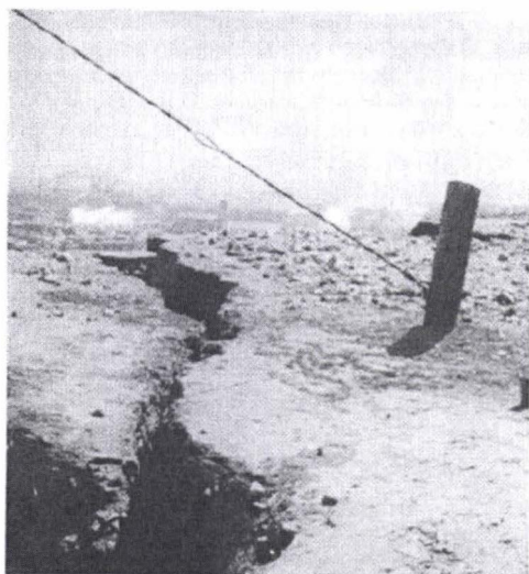
Fig. 9 – Fază activă a prăbușirii falezei.
