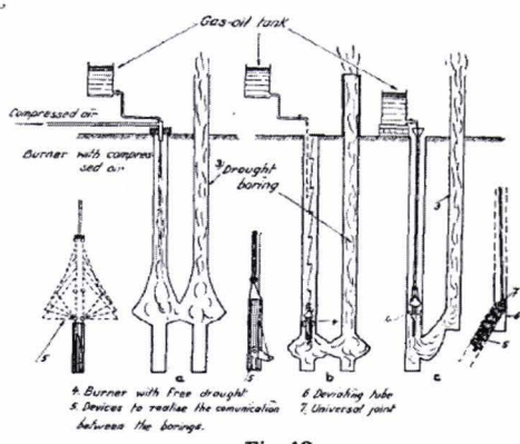
Fig. 17 – Tehnologia inovativă de stabilizare a solurilor argiloase prin ardere.
