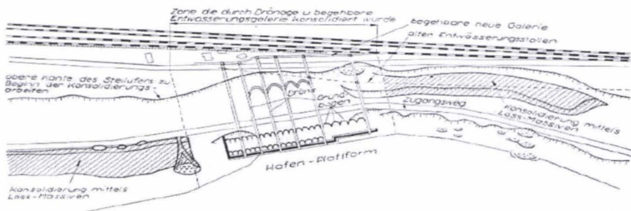
Fig. 13 – Schema lucrărilor la faleza spre port (sudică) din 1914-1934.
