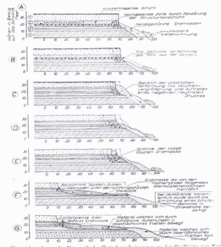
Fig. 8 – Mecanismul producerii alunecării și prăbușirii falezii.
