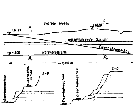
Fig. 3 – Decuparea falezii sudice prin linia CF
